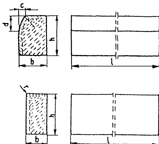
b) krawężnik rodzaju „b”
