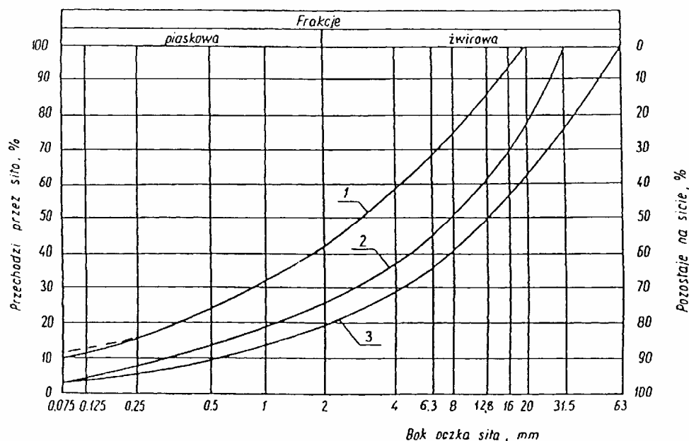
Rysunek 1. Pole dobrego uziarnienia kruszyw przeznaczonych na podbudowy wykonywane metodą stabilizacji mechanicznej 1-3 kruszywo na podbudowę pomocniczą (pobocza)
