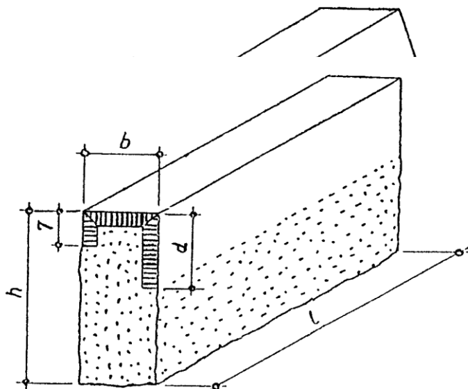
Rys. 1. Krawężnik uliczny odmiany UP, rodzaju A
