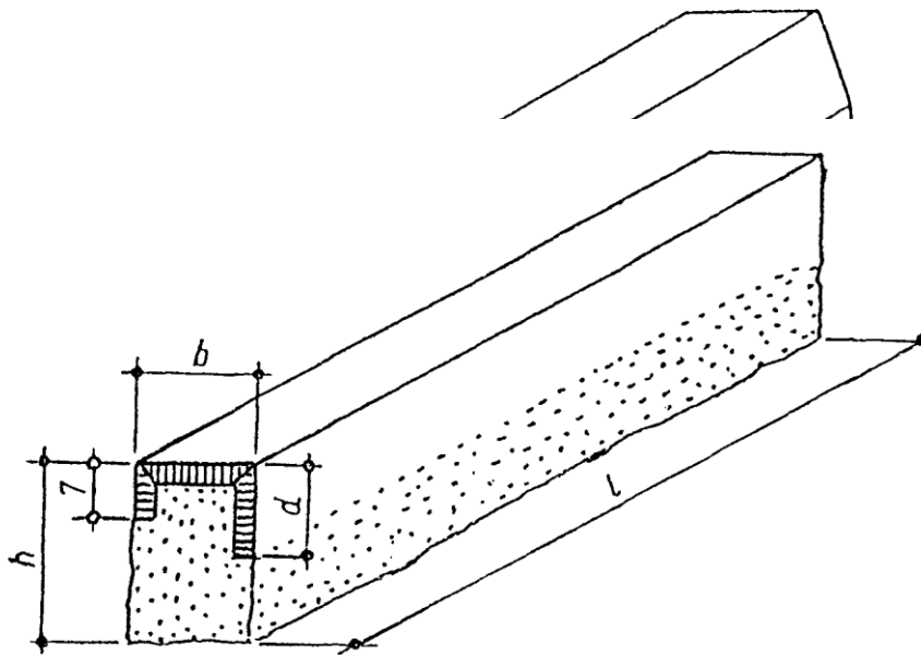
Tablica 3. Wymiary krawężników mostowych
