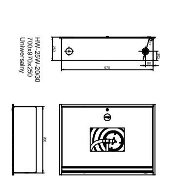
SCHEMAT SZAFKI HYDRANTOWEJ PODTYNKOWEJ
