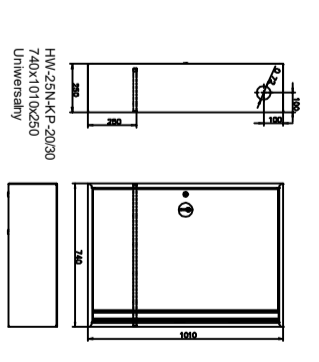
SCHEMAT SZAFKI NATYRKOWEJ
