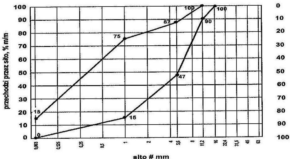
Rys. 1. Krzywe graniczne uziarnienia mieszanki kruszyw 0/11,2 mm do górnej warstwy podłoża ulepszanego
