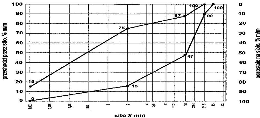
Rys. 4. Krzywe graniczne uziarnienia mieszanki kruszyw 0/31,5 mm do górnej warstwy podłoża ulepszanego
