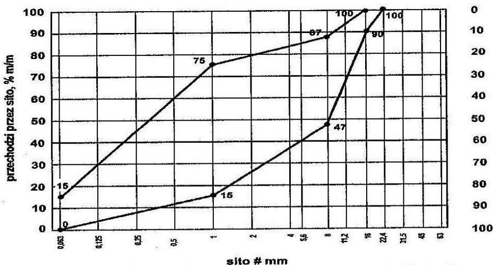
Rys. 2. Krzywe graniczne uziarnienia mieszanki kruszyw 0/16 mm do górnej warstwy podłoża ulepszanego
