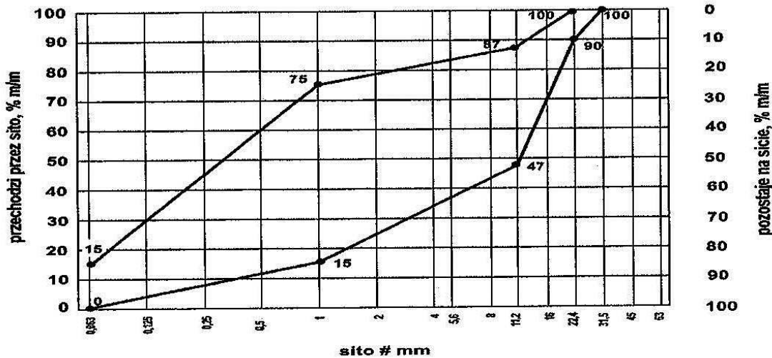
Rys. 3. Krzywe graniczne uziarnienia mieszanki kruszyw 0/22,4 mm do górnej warstwy podłoża ulepszanego
