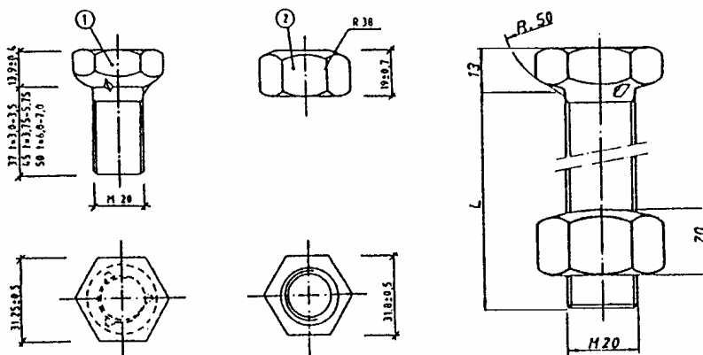
1 - śruba 2 - nakrętka
