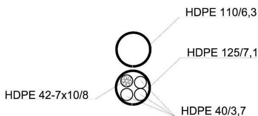
Rys.2 Profil kanału technologicznego KTP.
