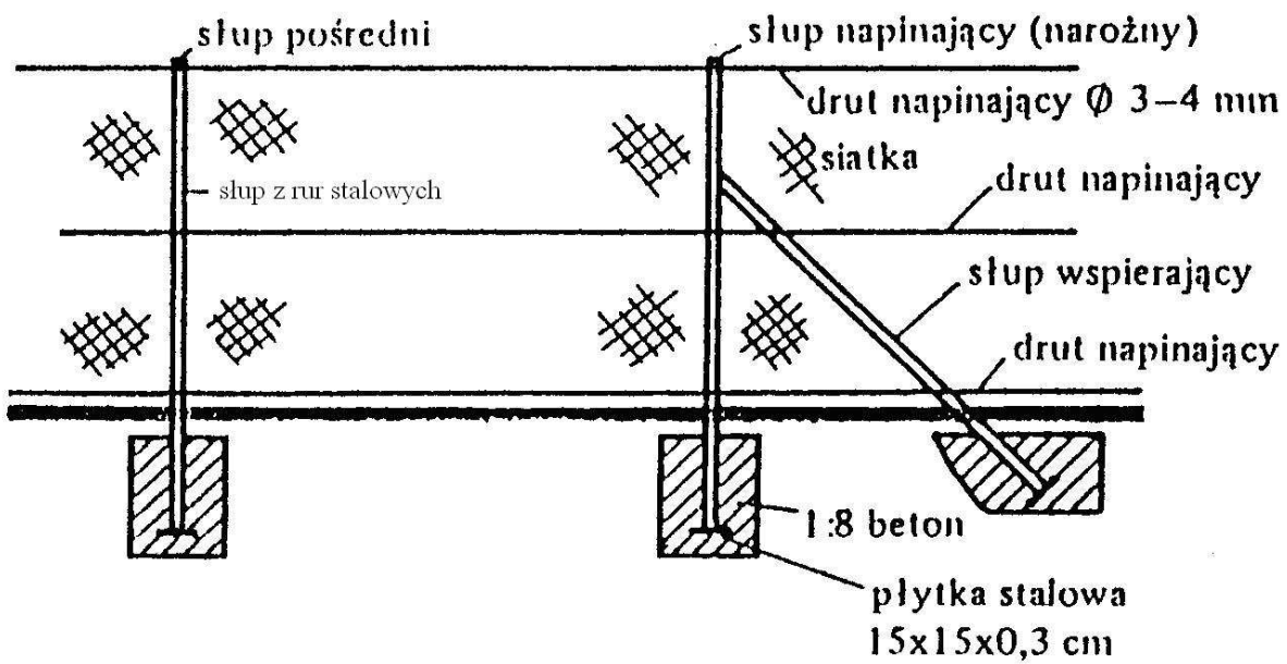
Rys. 3. Przykład wzmocnienia słupka narożnego lub słupka bramowego
