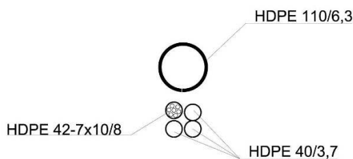
Rys.1 Profil kanału technologicznego KTu.
